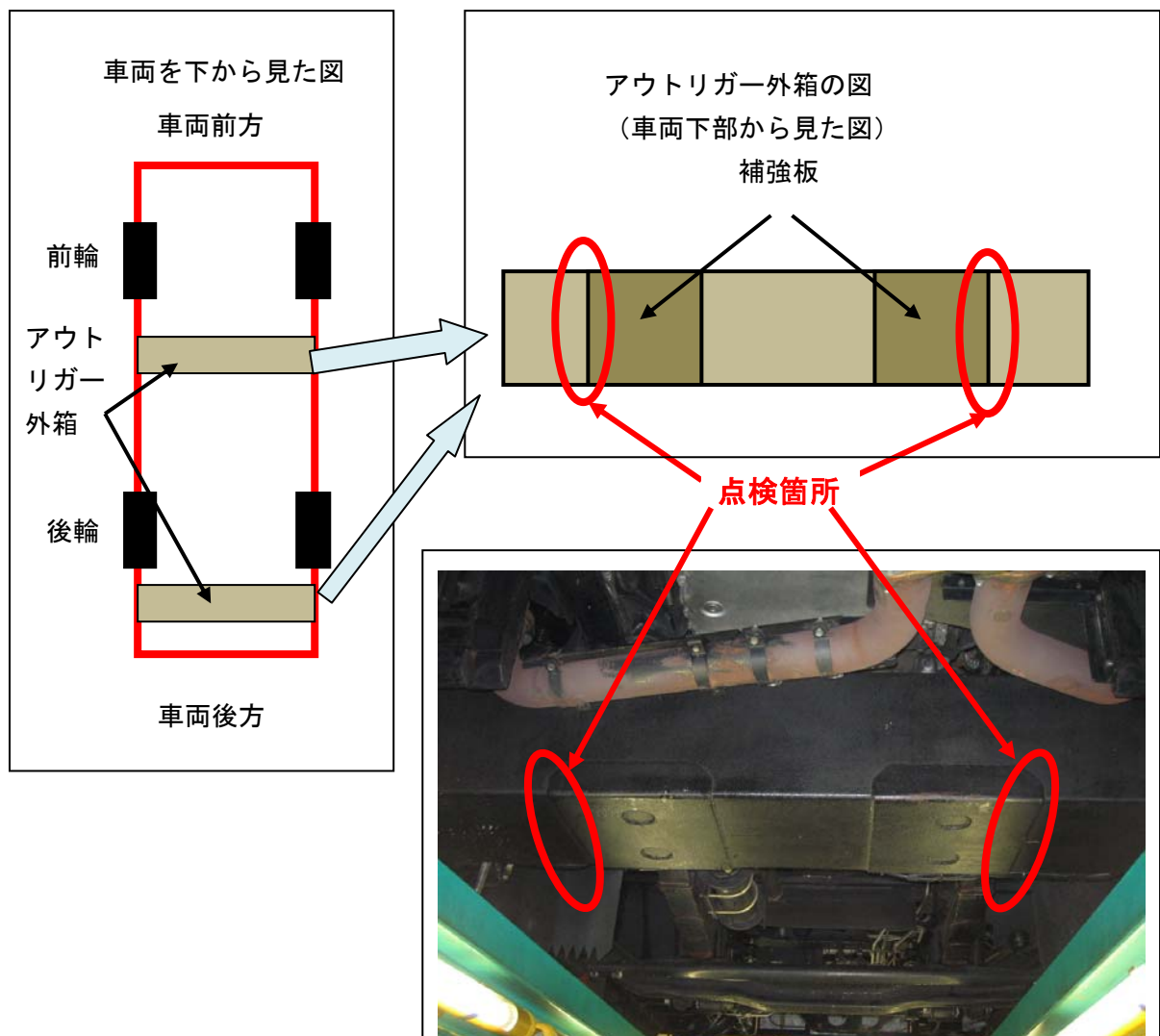
アウトリガー外箱の写真 (車両下部から見た写真)
